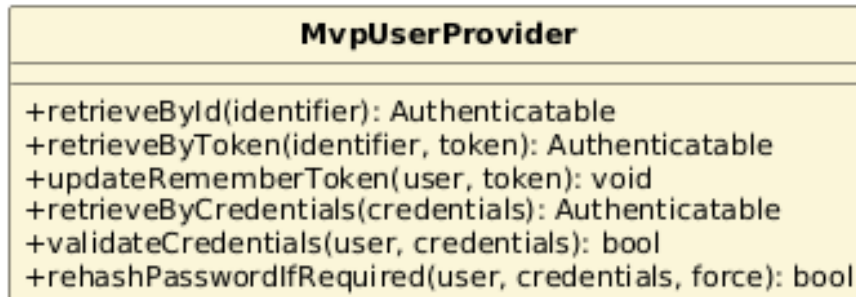
Figura 82: Classe — MvpUserProvider
